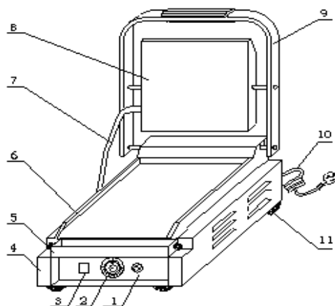
9—MANIGLIA DI LAVORO 10—CAVO DI ALIMENTAZIONE 11—PIEDI DI GOMMA
