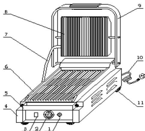
1—INDICATORE DI RISCALDAMENTO 2—REGOLATORE DI TEMPERATURA 3—INTERRUTTORE DI RETE 4—SCATOLA INFERIORE
